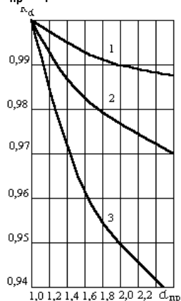
Рис. График определения K_a : 1,2,3 –соответственно все виды твёрдого топлива, жидкое и газообразное топливо
